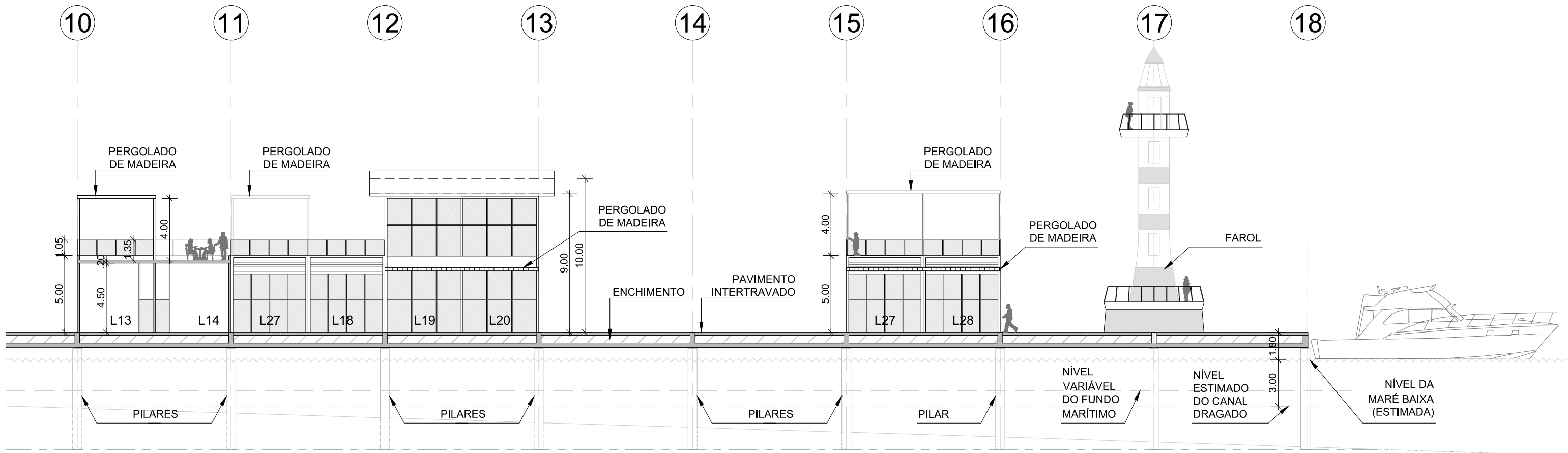
01 CORTE PARCIAL 03 EP ESCALA 1:250
